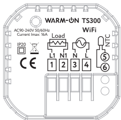
Schéma de câblage pour chauffage électrique
