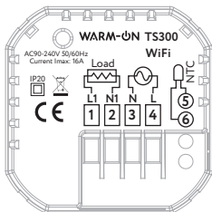
Verdrahtungsdiagramm für elektrische Heizung
